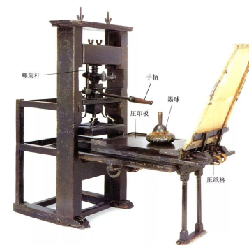
古腾堡印刷机
